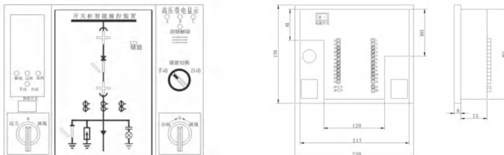
KLKZ-5产品外形（开孔）尺寸图
